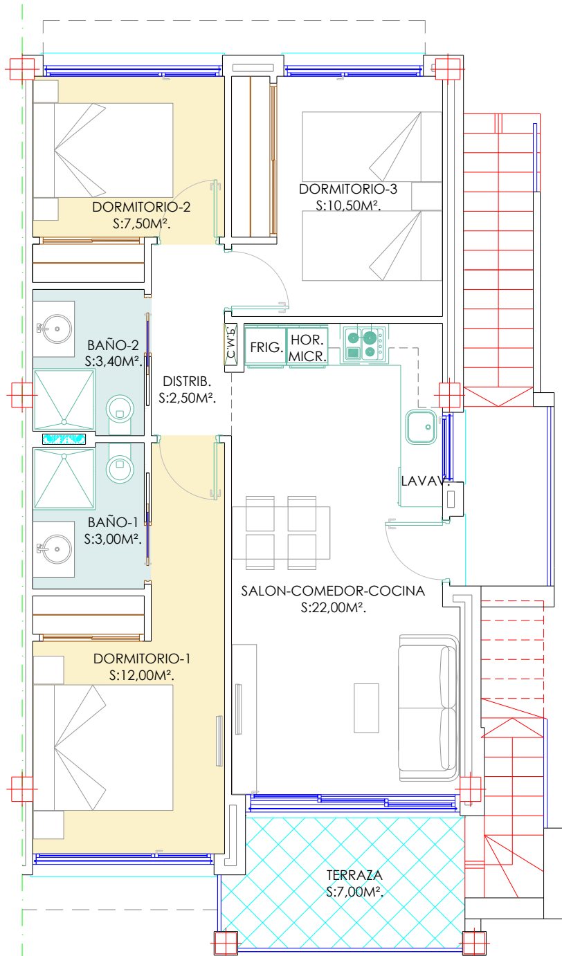
PLANTA PRIMERA
