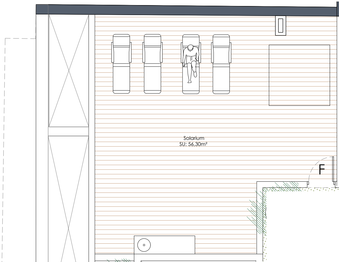
Planta Solarium
